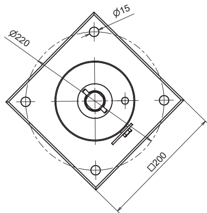
Rozměry spodní desky
