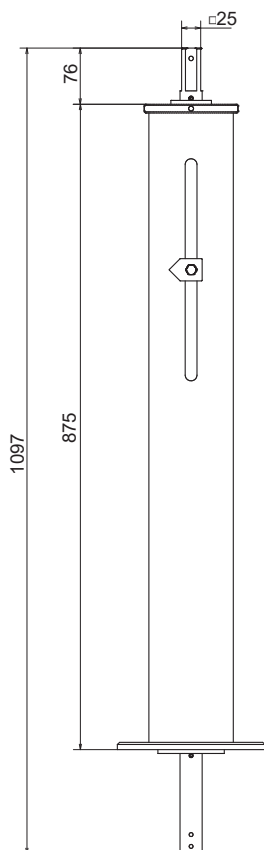
Rozměry sloupového stojanu
