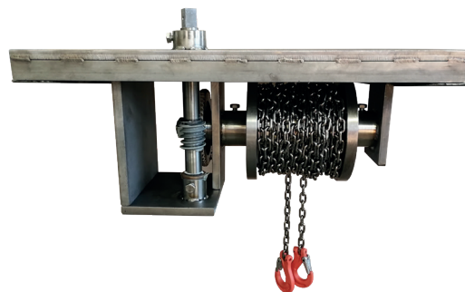
Zvedací zařízení pro koncové klapky určené pro připevnění hmoždinkami pod stropem. Příklad pro koncovou klapku DN 2800.
