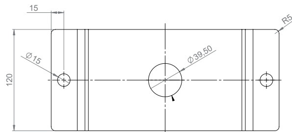
Rozměry stropního ložiska pro mřížový rošt se čtyřhranem nebo uzamykatelným krytem
