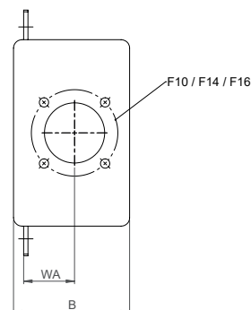
Anwendungsbeispiel mit aufgebautem Elektroantrieb
