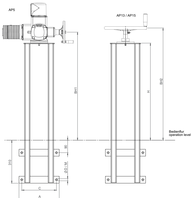
Anwendungsbeispiel mit aufgebautem Elektroantrieb
