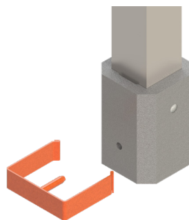
Klick-Pin
